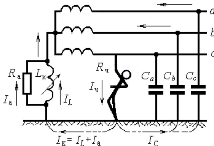
Рис. 11. Схема компенсации емкостного тока: L_K — компенсирующая катушка индуктивности; R_a — активное сопротивление катушки
